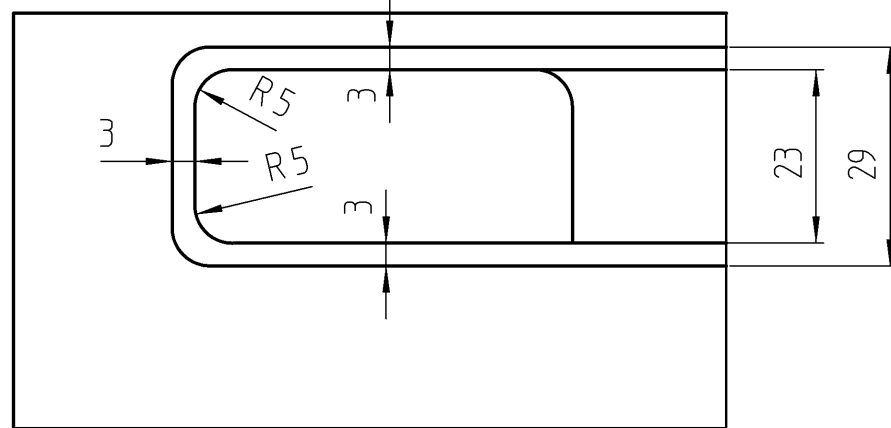
A-A 1:2
