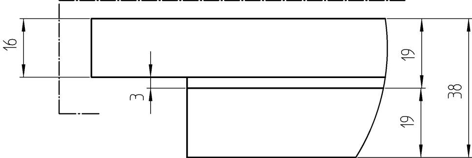
Detail1 1:1
