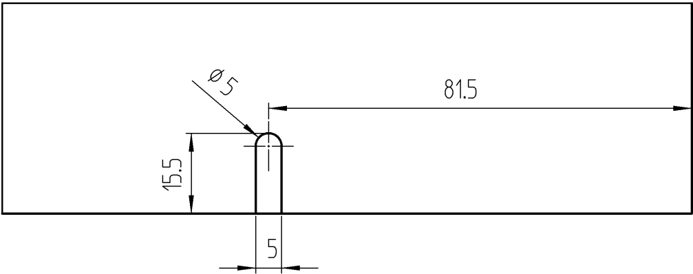
Detail1 1:1
